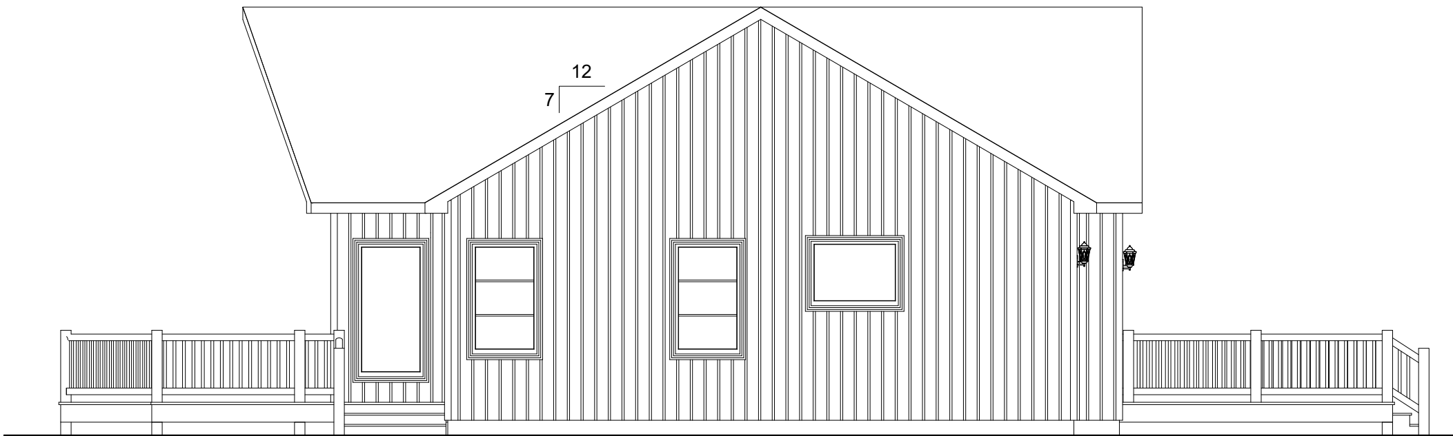
RIGHT ELEVATION
